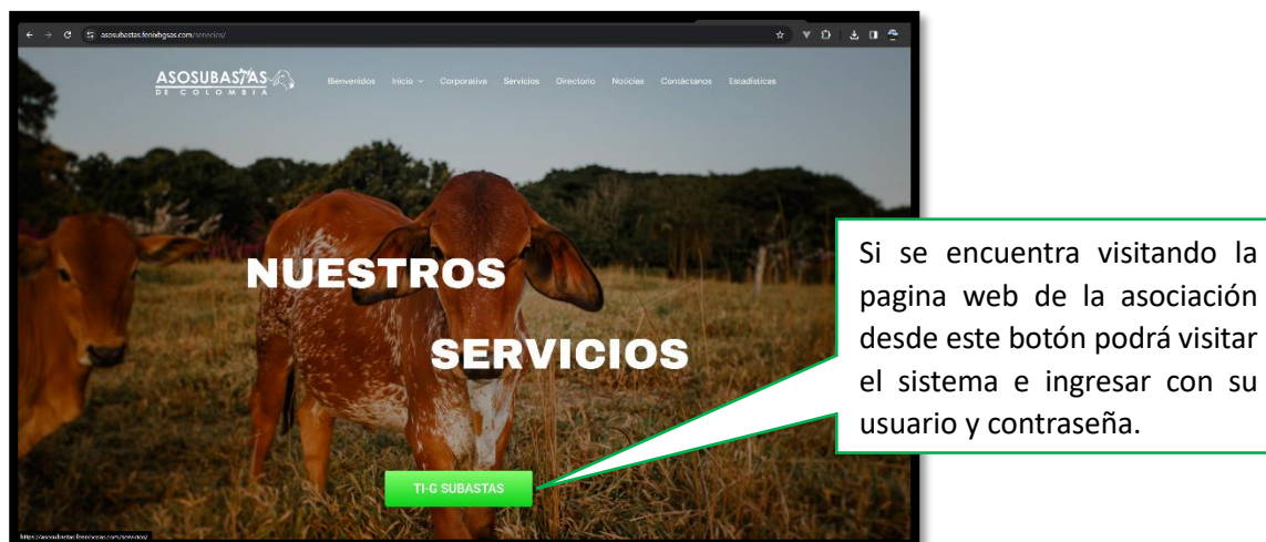
Figura 2 Pagina web-Servicios
